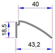
20mm'lik Alm. Eşik İç Profili AD16-080
