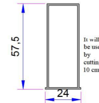
20mm'lik Alm. Eşik Sabit Kanat Yataklama Parçası AD16-083
